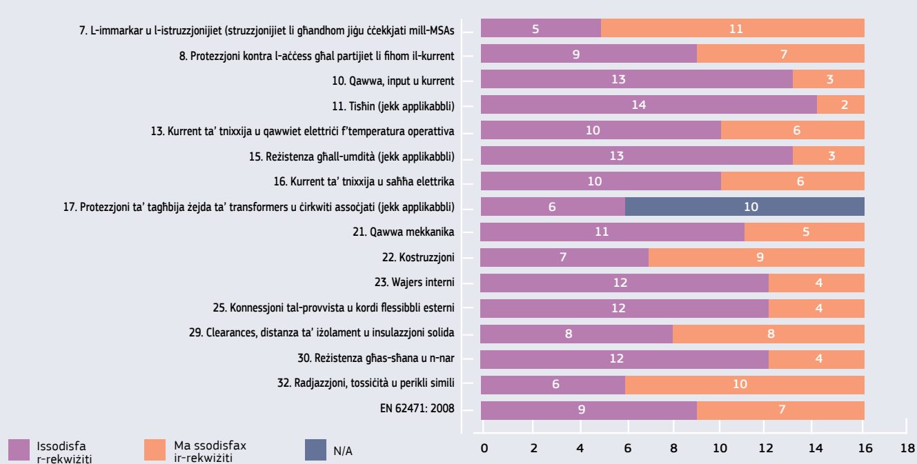
Figura 3 - Riżultati tat-test għal kull klawżola – EN 60335-1:2012 (N=16)
