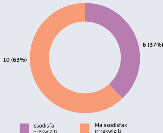
Figura 5 - Riżultati, EN 60335-2-109:2010 – Klawżola 32 Radjazzjoni, tossiċità u perikli simili (N=16)
