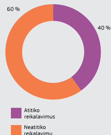
Suaugusiesiems skirtų dviratininkų šalms padirbiniai. Šoninio susidūrimo / sukimosi bandymai (N=5)
