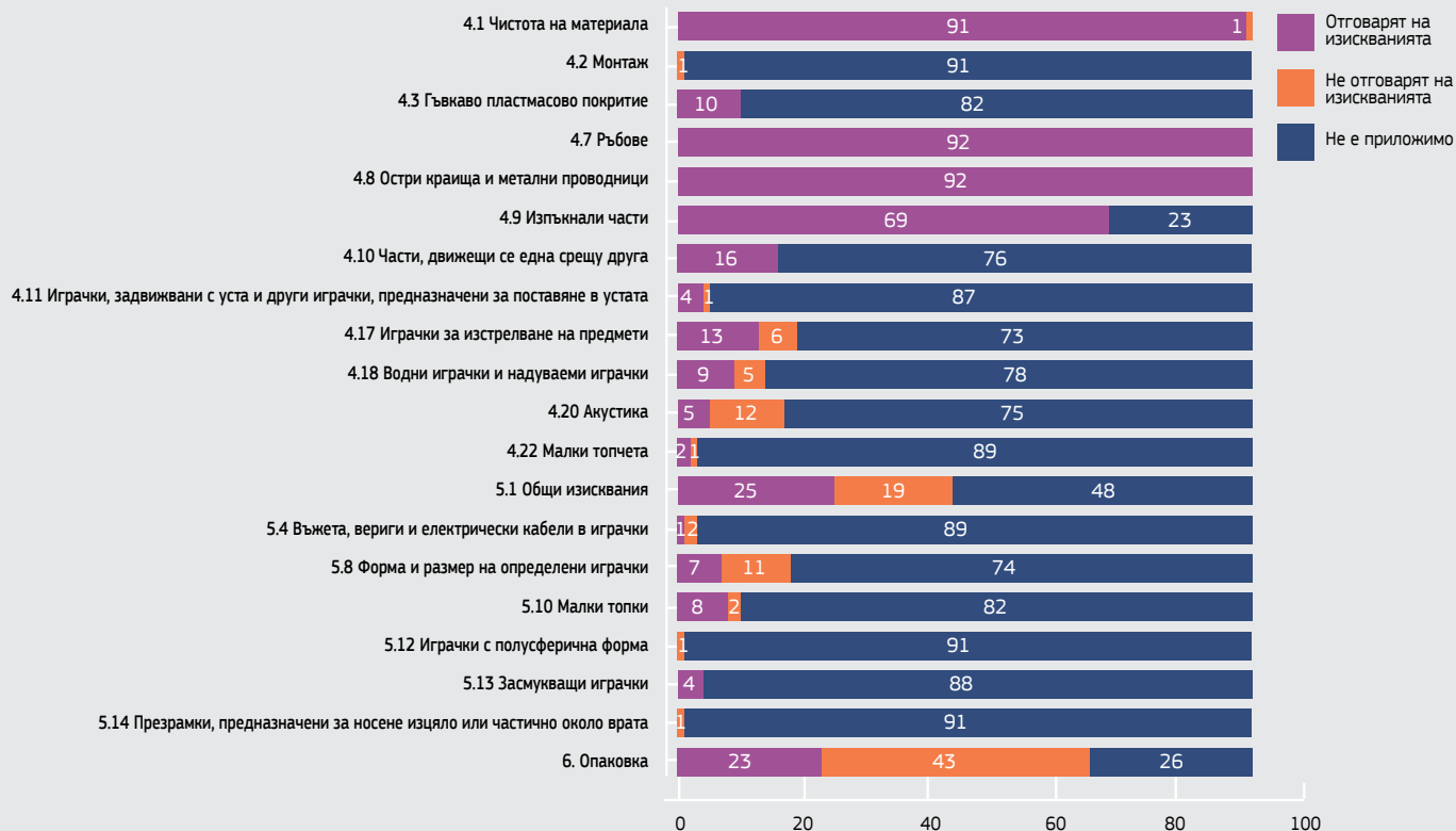
Фигура 4 — Резултати от изпитването по клаузи — EN 71-1:2014+A1:2018 (N=92)
